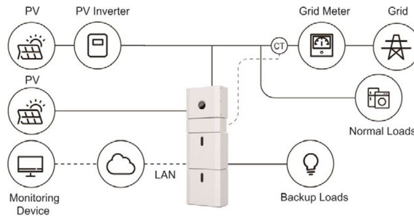
Figura 3 Sistema di accumulo ibrido accoppiato
