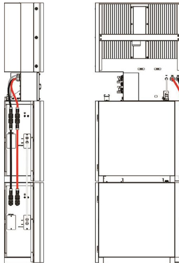
Figura 29 Cablaggio del cavo di alimentazione della batteria
