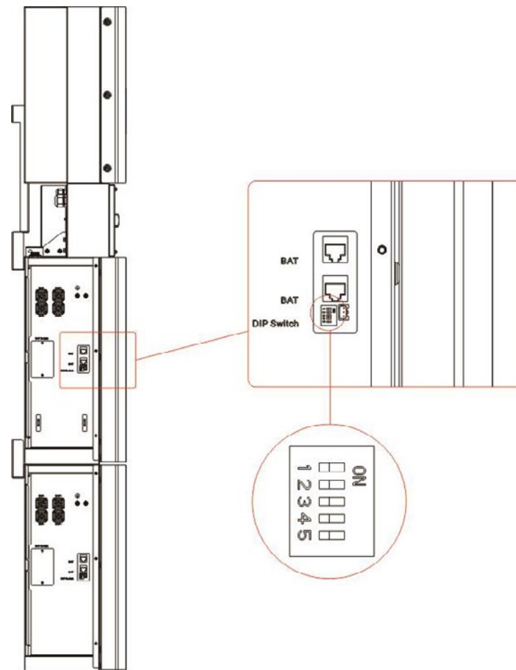
Figura 32 Interruttore DIP
