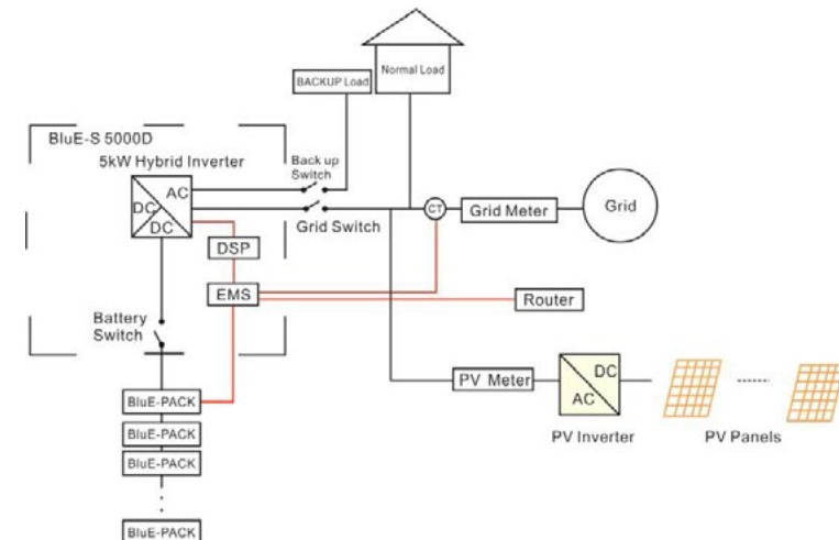
Figura 38 Sistema ad accoppiamento CA
