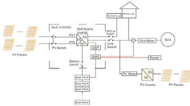
Figura 39 Sistema ad accoppiamento ibrido
