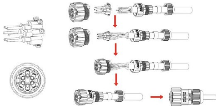
Figura 36 Connettore DRM
