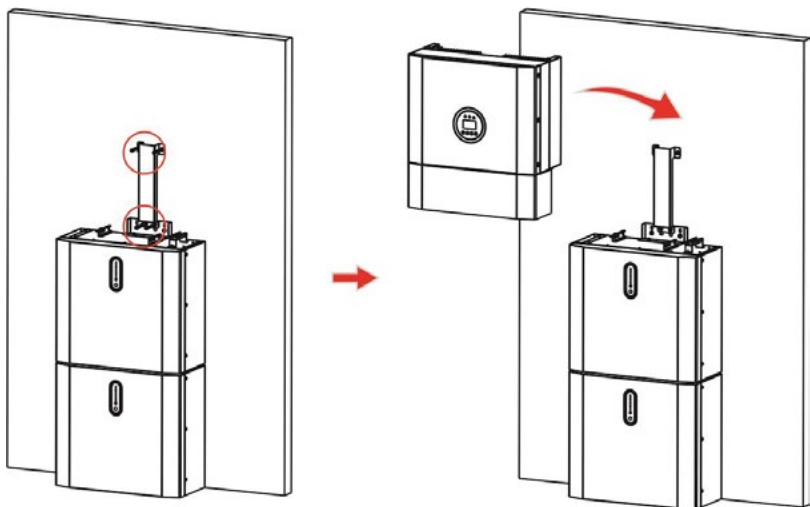
Figura 22 Installazione dell'inverter
