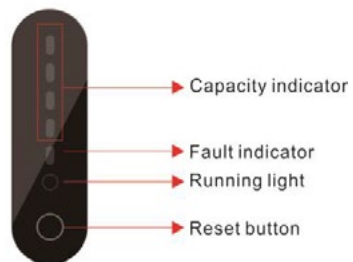
Figura 42 Interfaccia del pacco batteria
